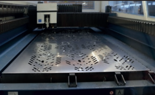
Im zweiten Schritt werden die Segmente separiert
