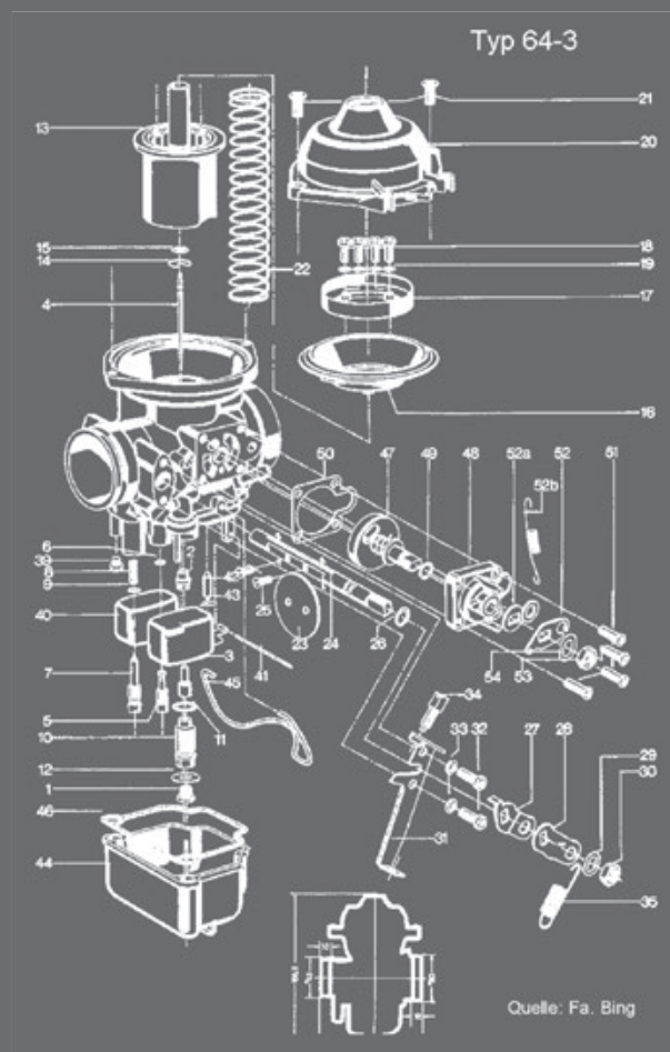
Leerlaufgemischschraube (7) ganz vorsichtig bis zum Anschlag hineinschrauben.
