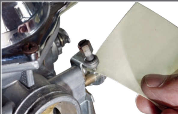
Drosselklappenanschlagschraube (34) so weit hineindreihen, bis das Papier sich gerade noch zerstörungsfrei herausziehen lässt.
